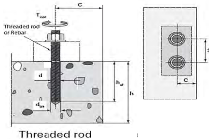
FIGURE 1—INSTALLATION PARAMETERS
